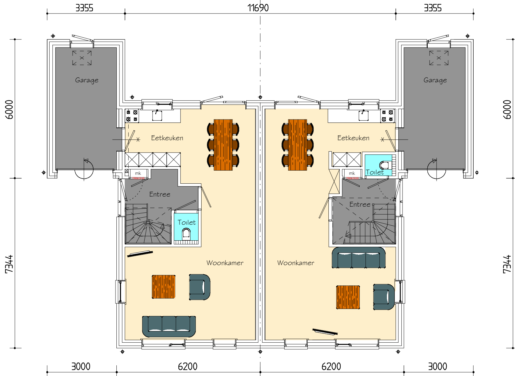
Beganegrond
